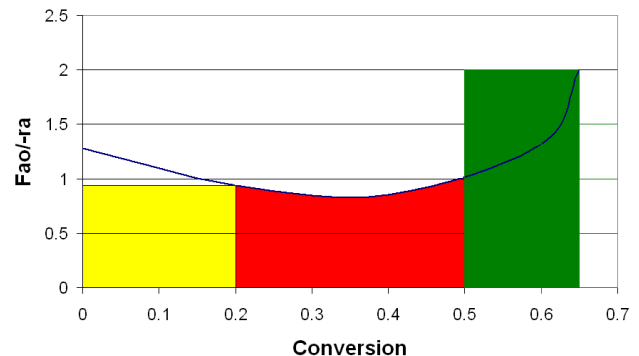
Levenspiel Plot
